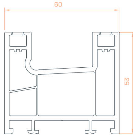
60'lık Sürme Kasa Profili 60 mm Sliding Frame Profile
