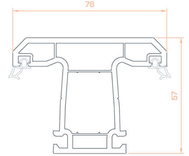
Sürme Orta Kayıt Profili / Corner Turn Pipe
