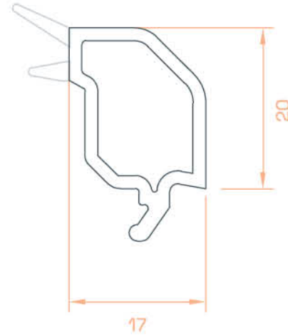
60'lık Çift Cam Çıta 60 mm Double Glazing Bead
