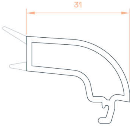
60'lık Tek Cam Çıta 60 mm Single Glazing Bead
