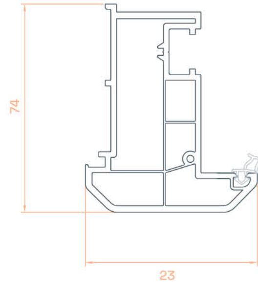
Hareketli Orta Kayıt Moving Central Profile
