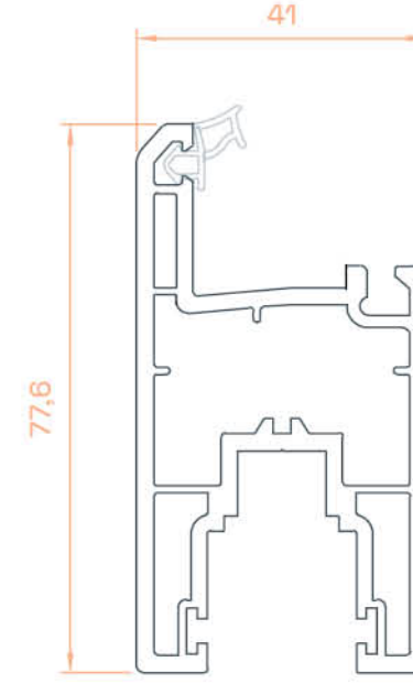
60'lık Sürme Kanat Profili 60 mm Sliding Sash Profile
