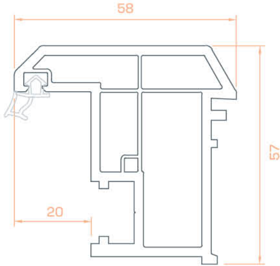
Hareketli Orta Kayıt Moving Central Profile
