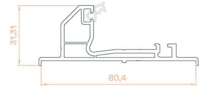
Sürme Kilitleme Profili Sliding Lock Profile
