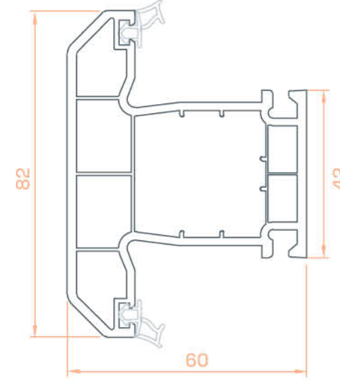
Orta Kayıt Profili / Middle Supporter Profile
