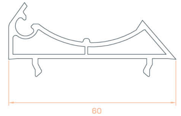
Köşe Dönüş Adaptörü Corner Turn Adapter
