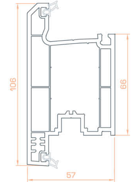
Dışa Açılan Kapı / Outward Opening Door
