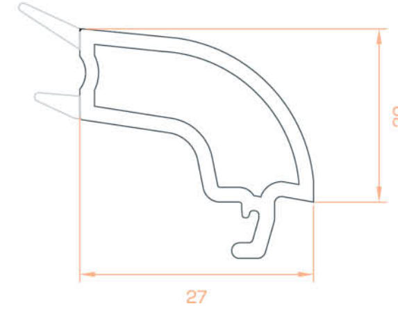
24'lık Cam Çıta (72'lik) 24 mm Glazing Bead (72 mm)
