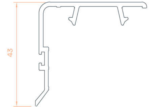
Alın Kapama / Edge Closure
