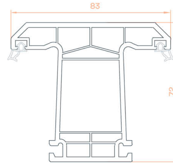
Orta Kayıt Profili / Middle Supporter Profile
